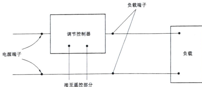
图 5 信号和控制器的测量布置
