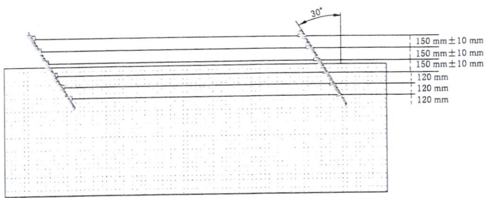
图 A.3 实体围墙 6 线斜装效果图
