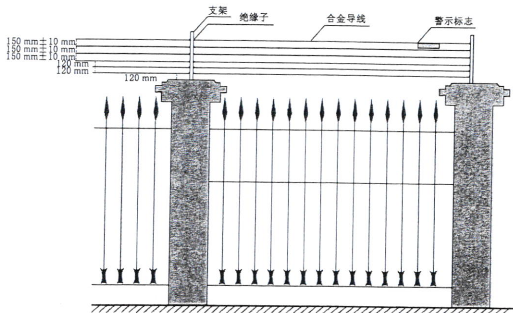
图 A.2 栅栏围墙安装示例
