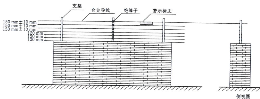
图 A.1 实体围墙上安装示例
